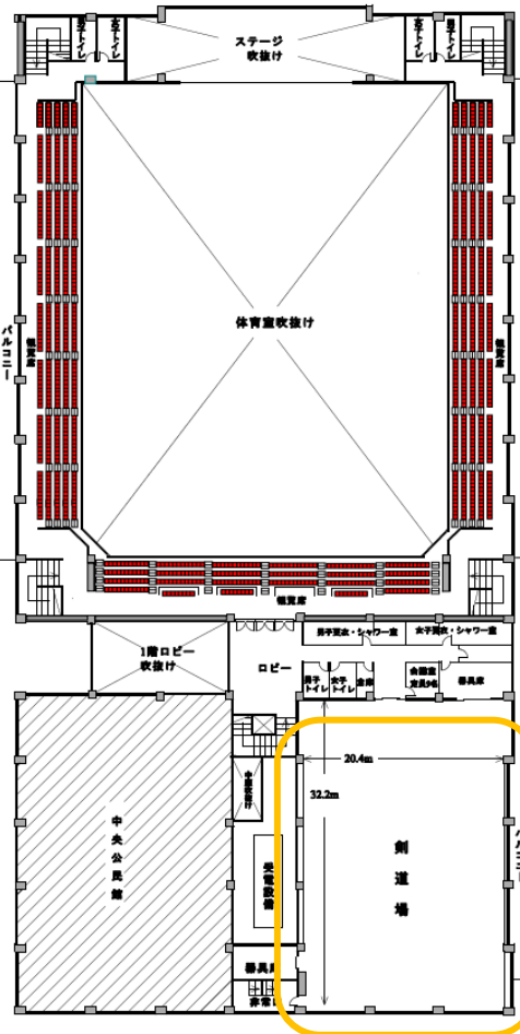
宮崎市総合体育館 二階 平面図
